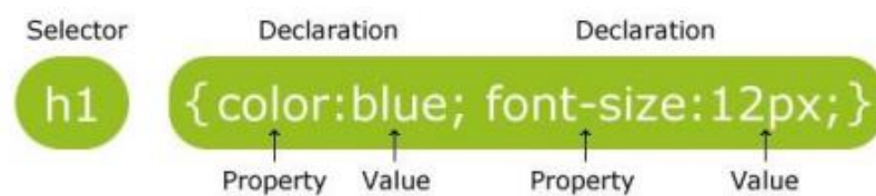
Gambar 4-1. Penulisan CSS
